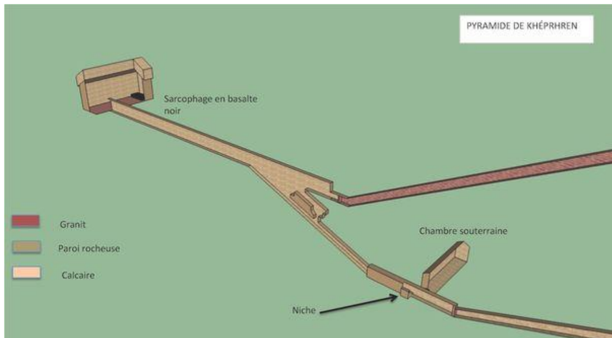
Vue axonométrique de la pyramide.
